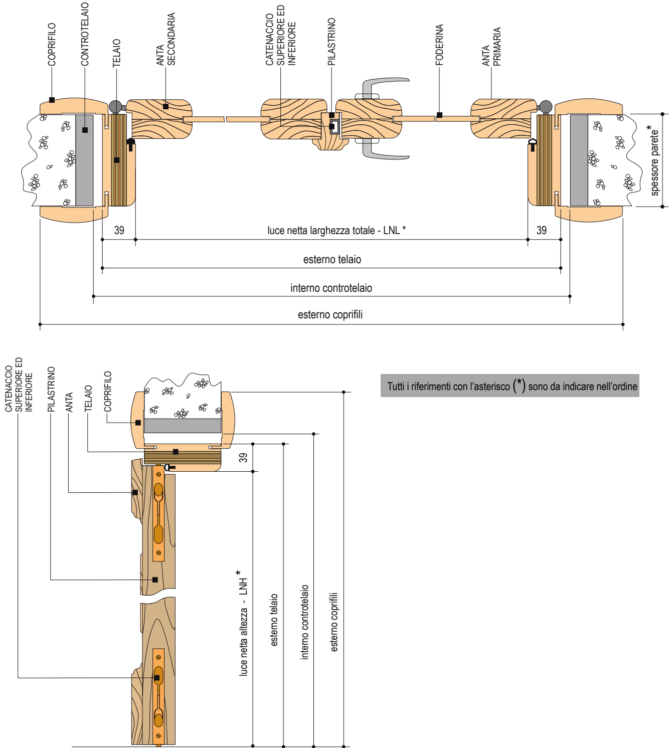
CARATTERISTICHE DIMENSIONALI
