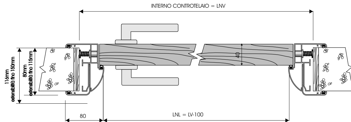
definizione delle misure da sezione longitudinale
