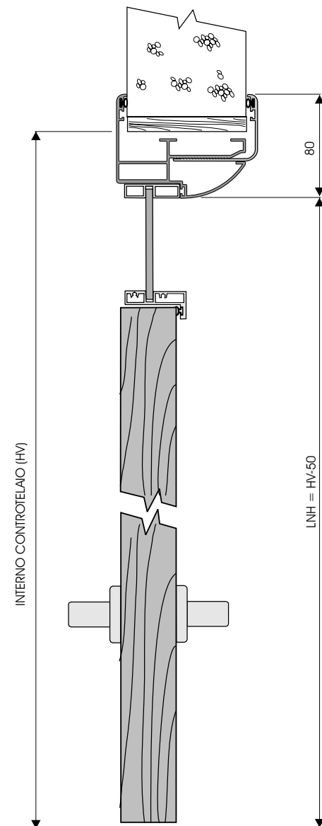
definizione delle misure da sezione longitudinale
