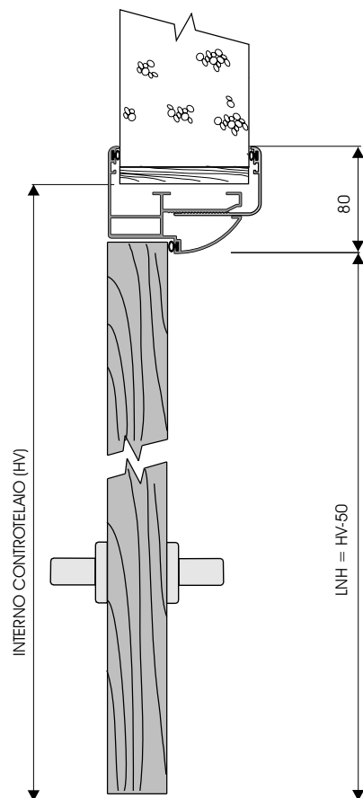
definizione delle misure da sezione longitudinale
